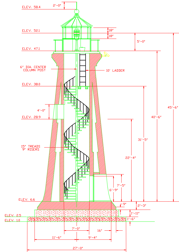
SECTION D-D
